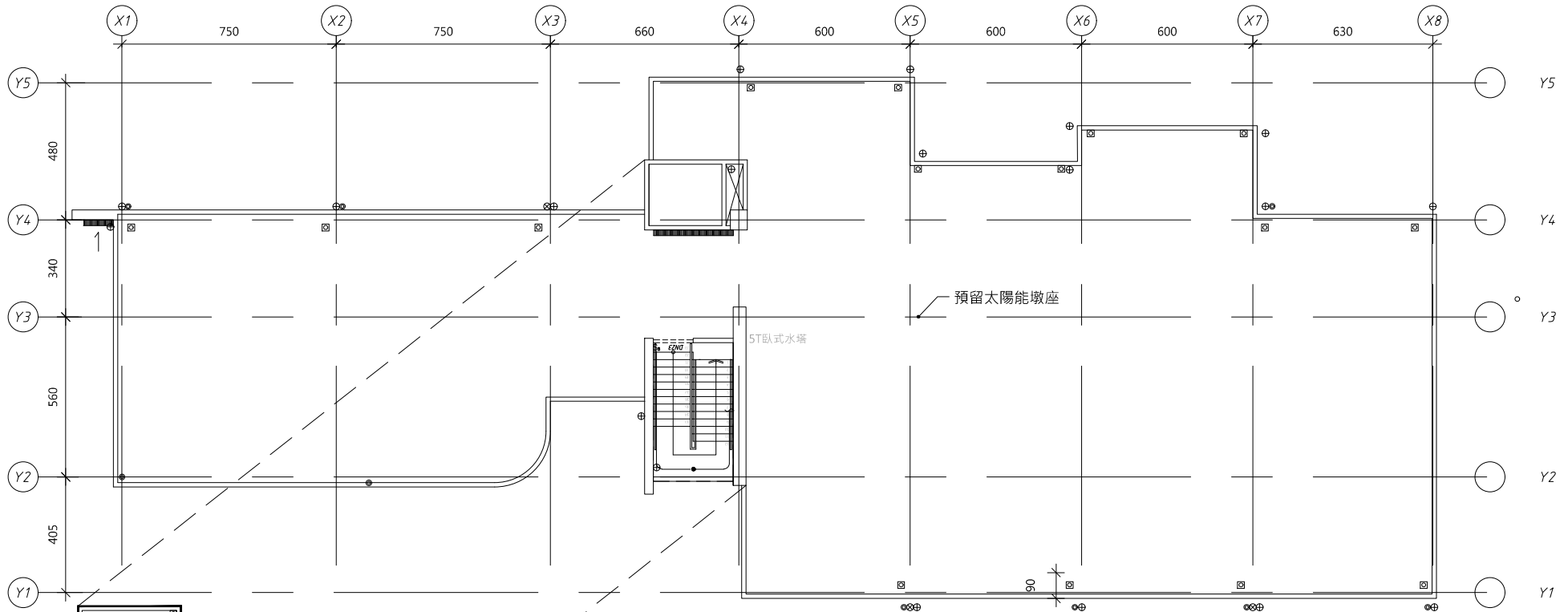
屋突層平面圖
